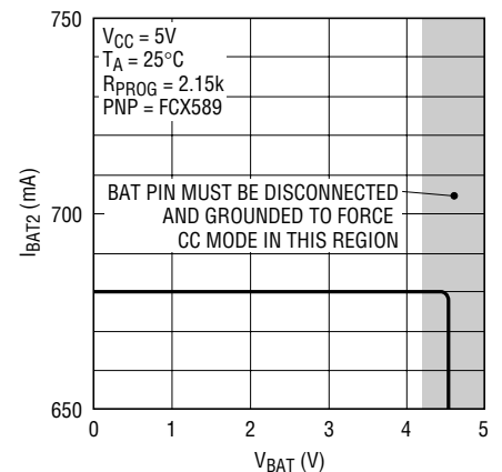
I_{BAT2} vs V_{BAT}
