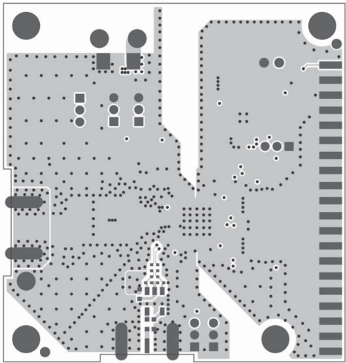
Bottom Side
