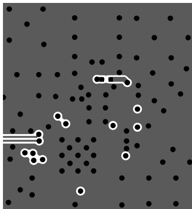
Bottom Side
