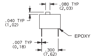
BD08E SPST
