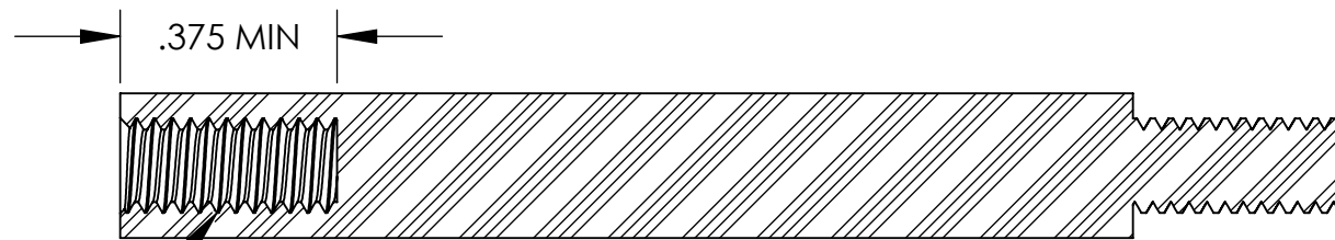
SECTION A-A
