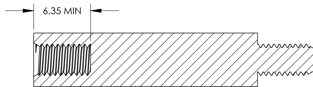
SECTION A-A
