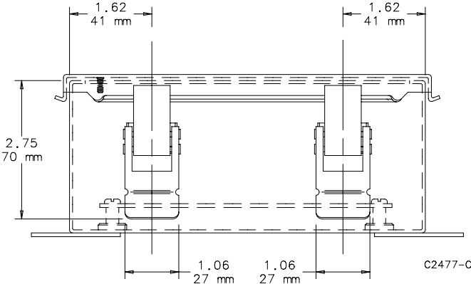
A ≥ 8.00 (203mm)
