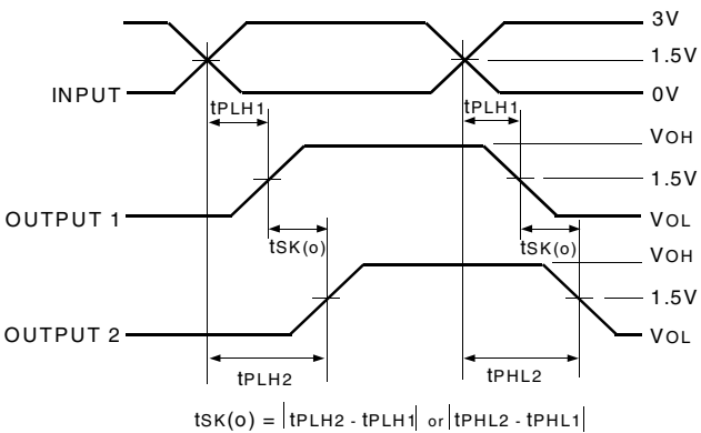
Output Skew
