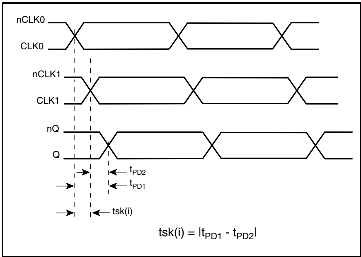
Input Skew
