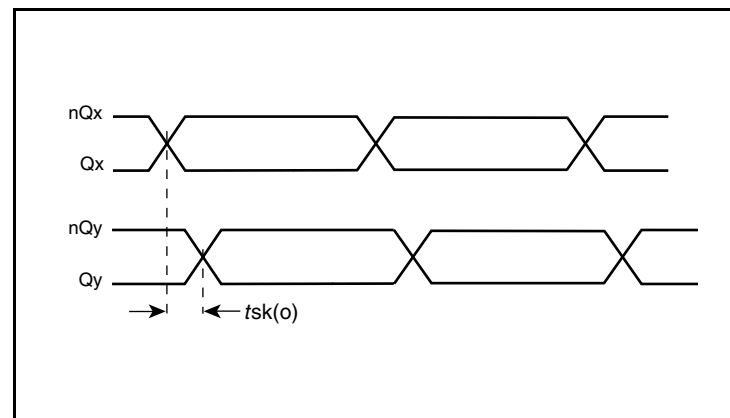
Output Skew
