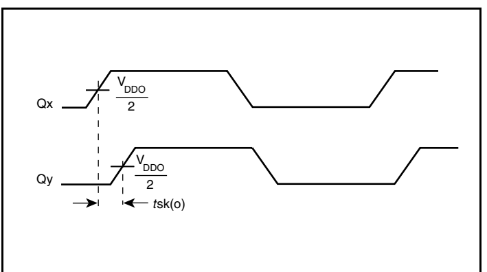
Output Skew
