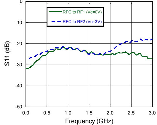
RF1 Return Loss
