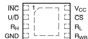
TDFN (VP2)
