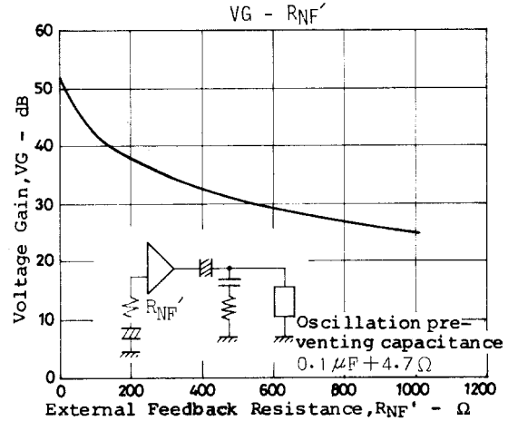
Figure 20. V_G - R_{NF'}
