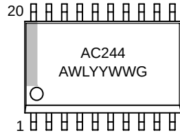
SOIC-20W
