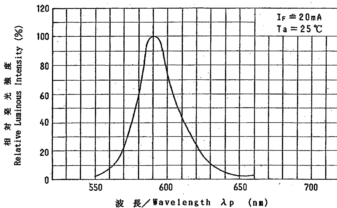
相对発光強度 - 波長特性 Relative Luminous Intensity Wavelength Characteristics
