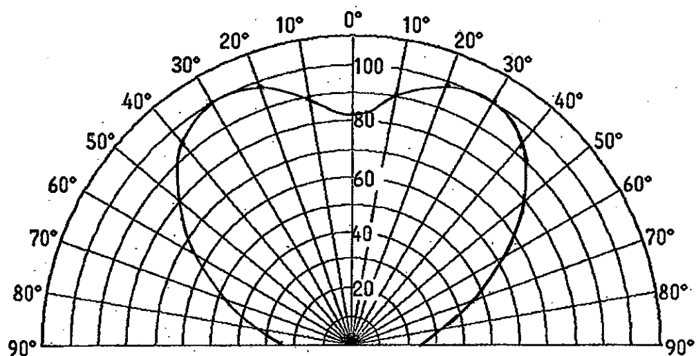
相对発光強度 Relative Luminous Intensity (%)
