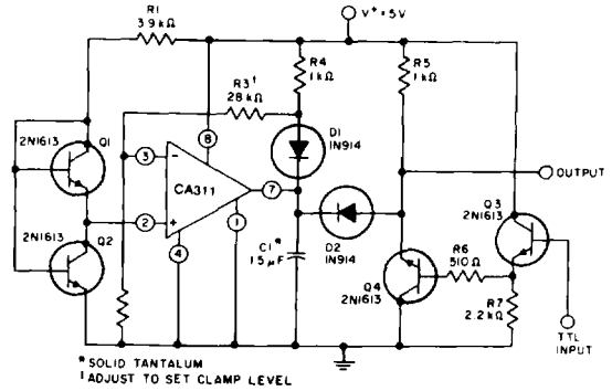
Fig. 31 - Precision squarer.
