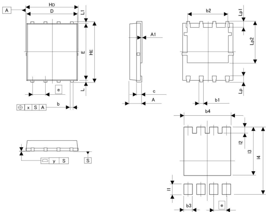
HSOP8 ( 5 x 6 )
