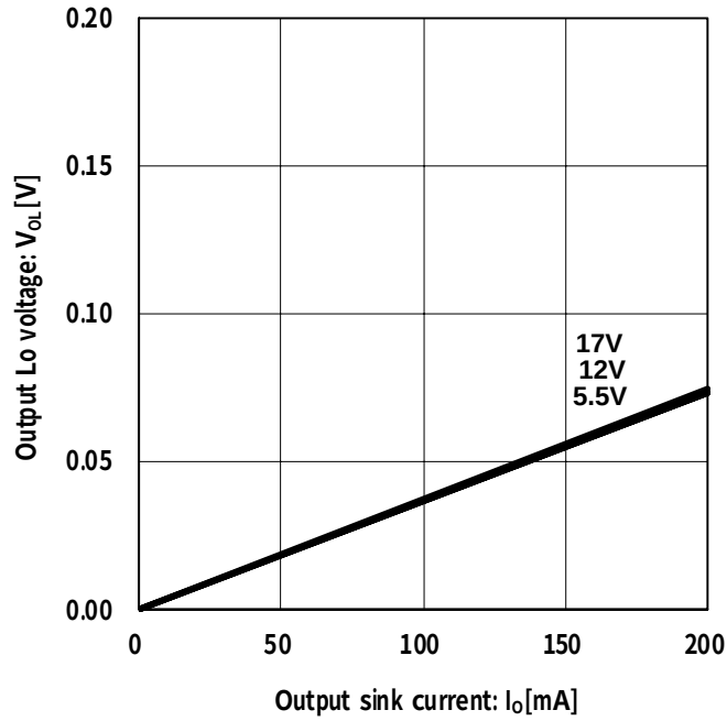
Fig. 20 Output Lo voltage ( T_a=25^{\circ}C )
