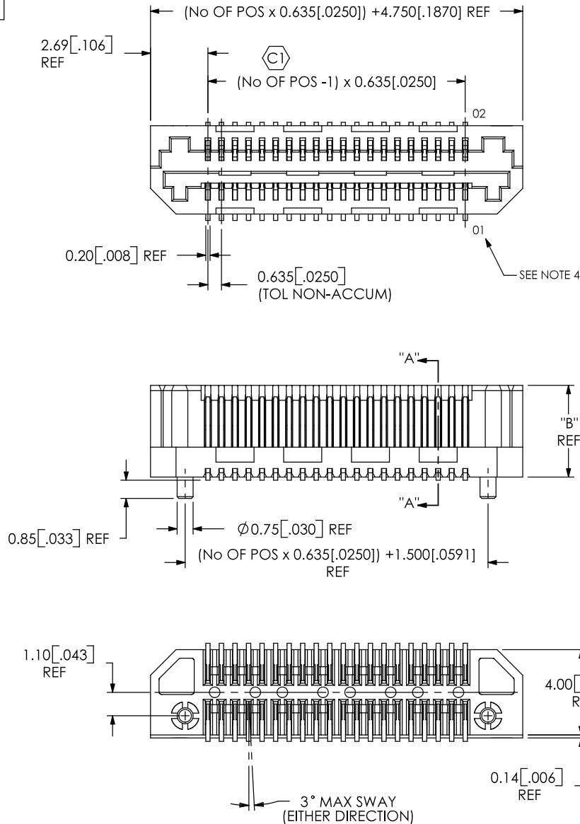
FIG. 1 LSS-120-01-X-DV-A SHOWN
