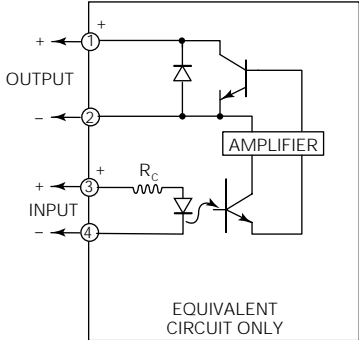
ODC Operating Diagram
