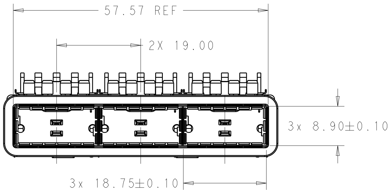
SCALE 2:1
