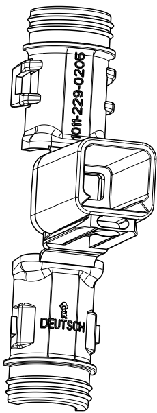
SCALE 1:1 Maßstab
