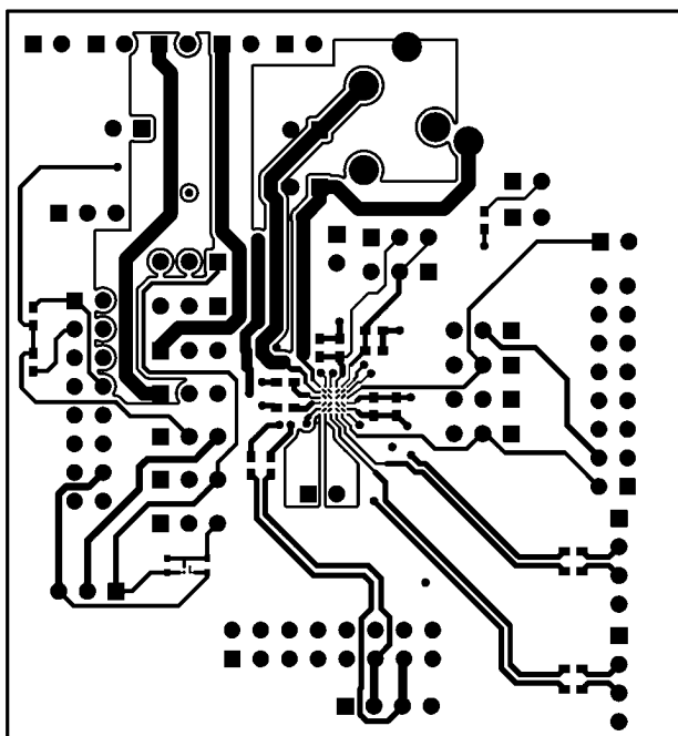
FIGURE 29. Top Layer
