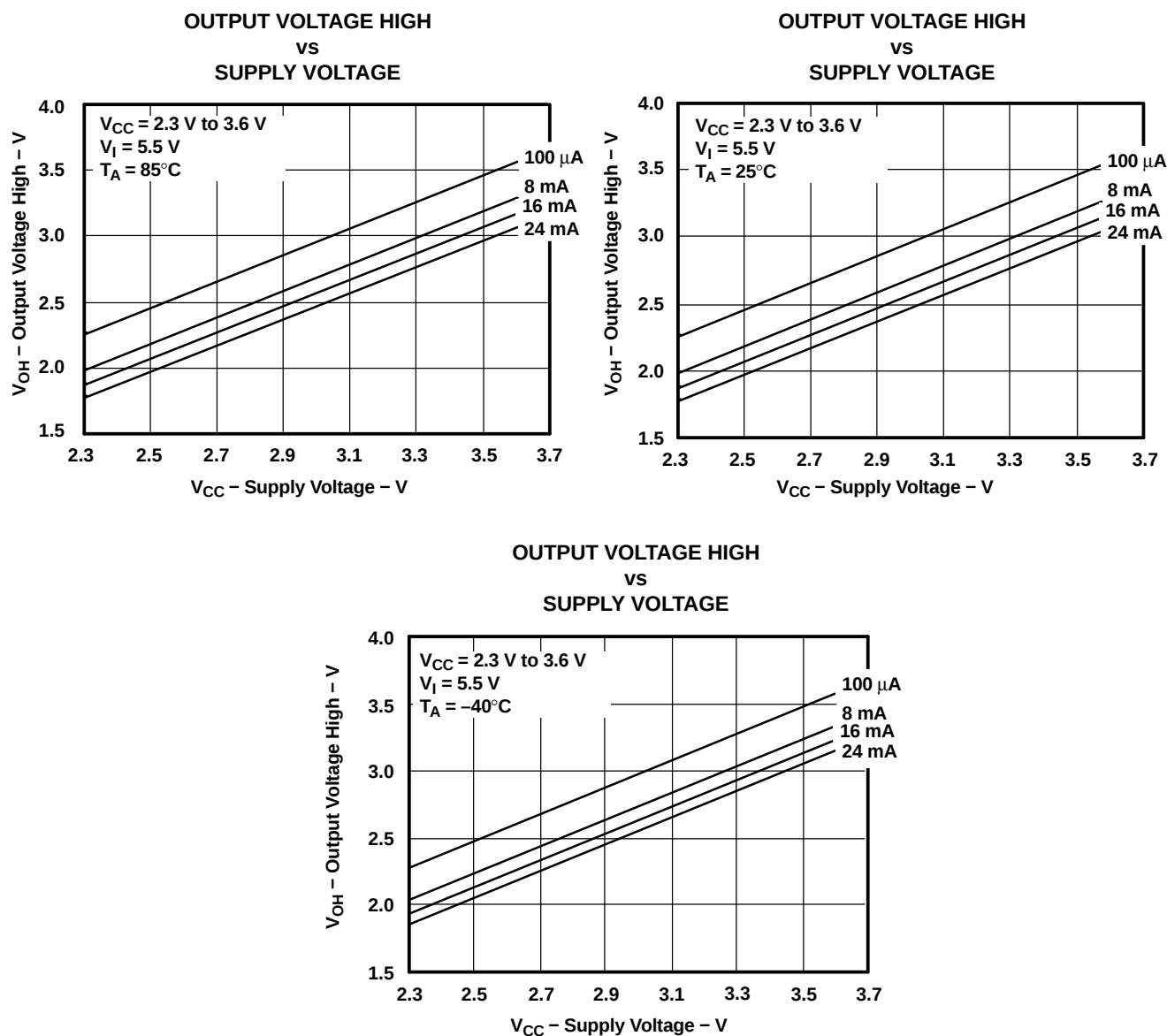
Figure 4. V_{OH} Values
