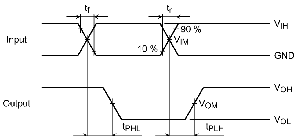
Fig. 11.8.1 t_{PLH}, t_{PHL}
