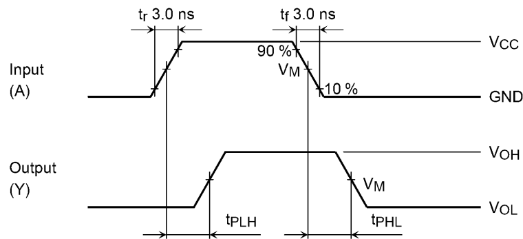
Fig. 9.6.1 tPLH, tPHL
