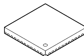
QFN48-P-0707-0.50
