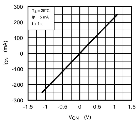
Fig. 14.4 I_{ON} - V_{ON}
