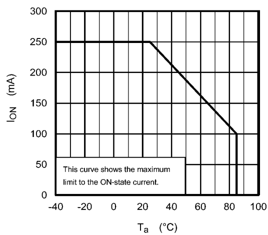
Fig. 14.2 I_{ON} - T_a
