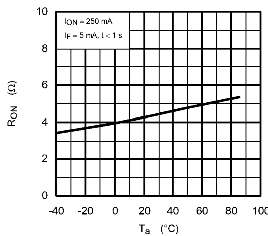
Fig. 14.5 R_{ON} - T_a
