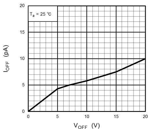
Fig. 12.9 I_{OFF} - V_{OFF}
