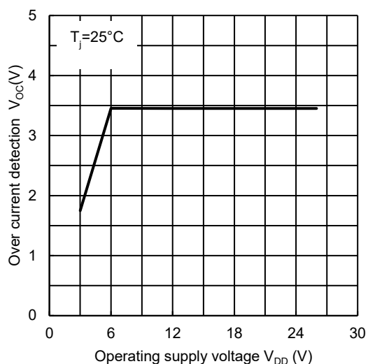
V_{OC} - V_{DD}
