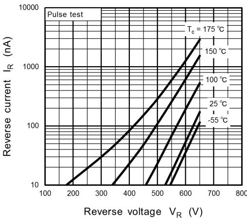
Fig. 9.3 I_R - V_R
