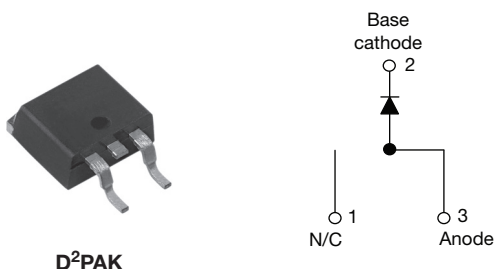
D²PAK
