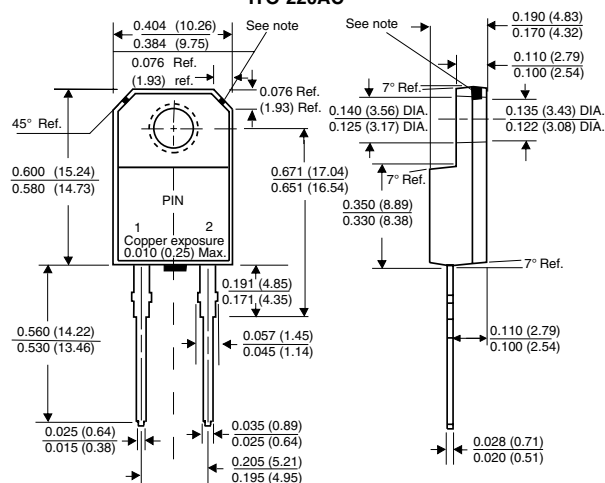
ITO-220AC
